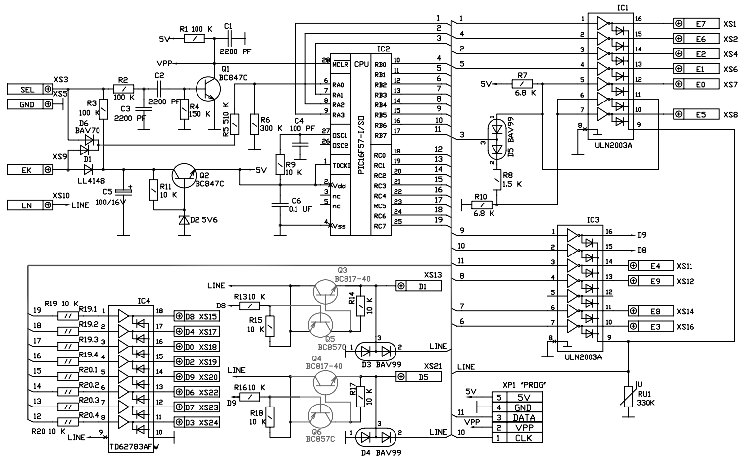
БК-100М Схема электрическая принципиальная
